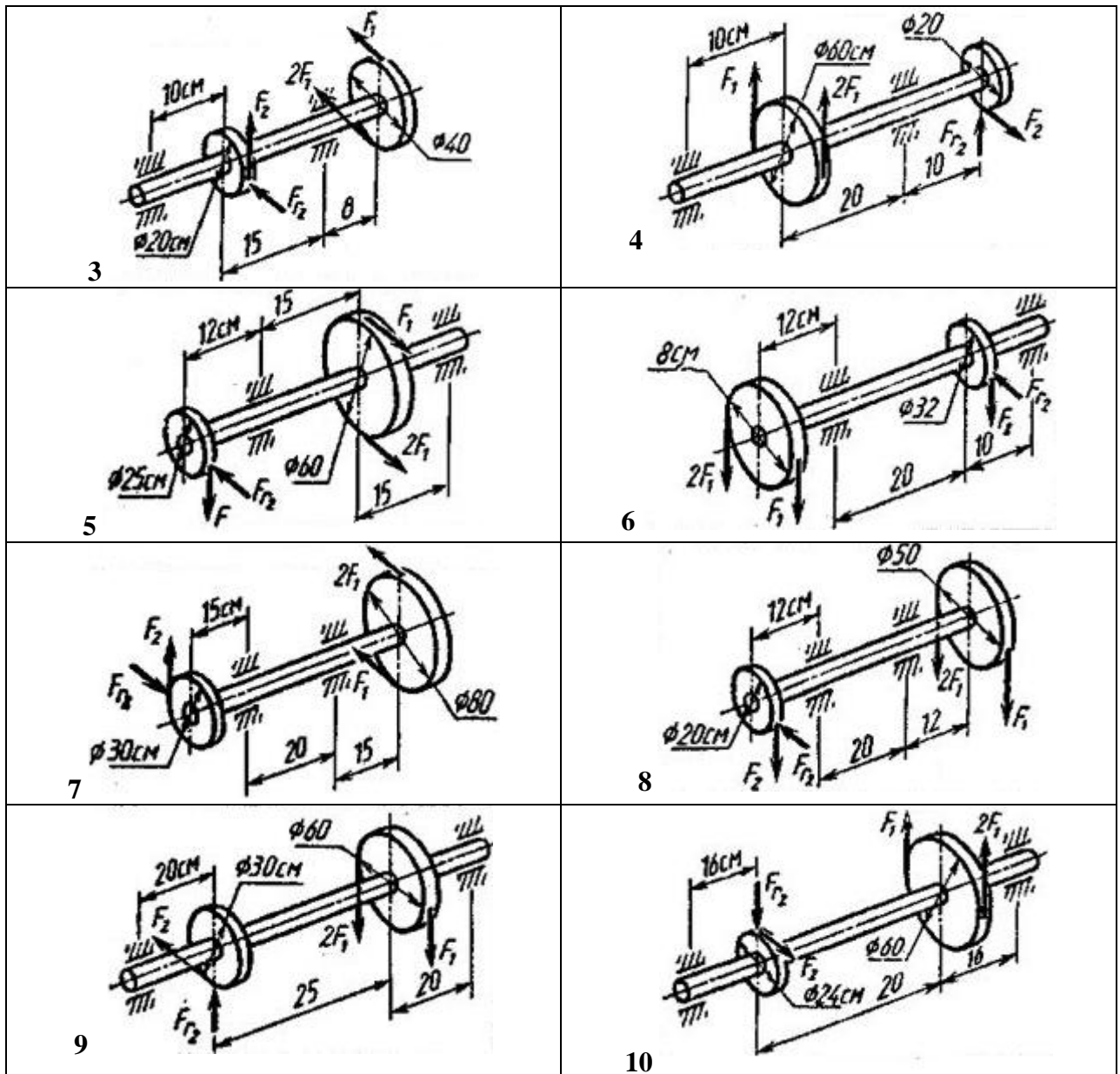
Рис. 5 - Схема задачи
