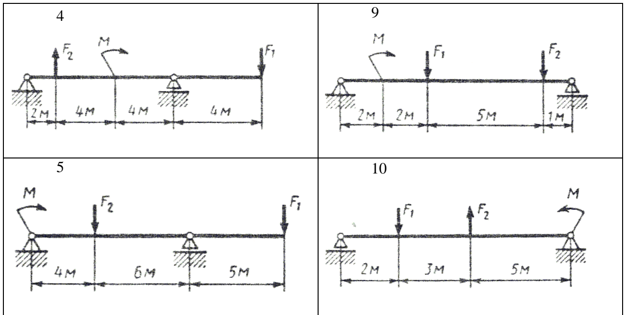
Рис. 12 - Схема задачи
