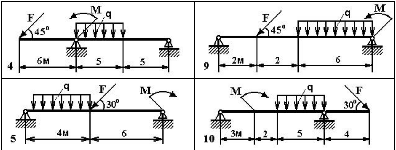
Рис. 4 - Схема задачи
