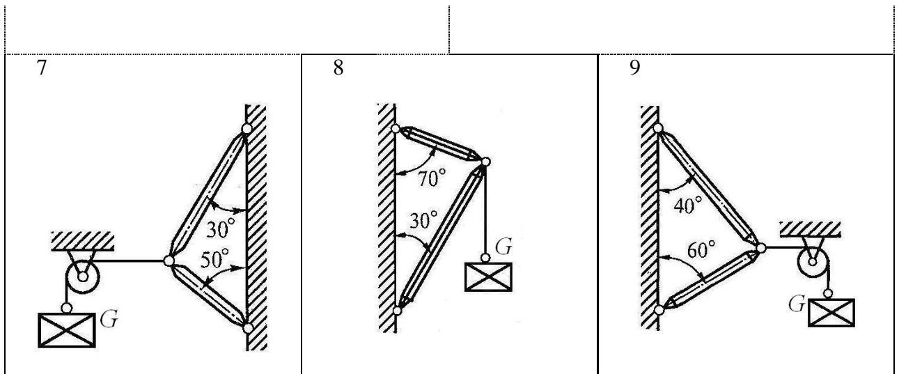
Рис. 1 – Схемы задач
