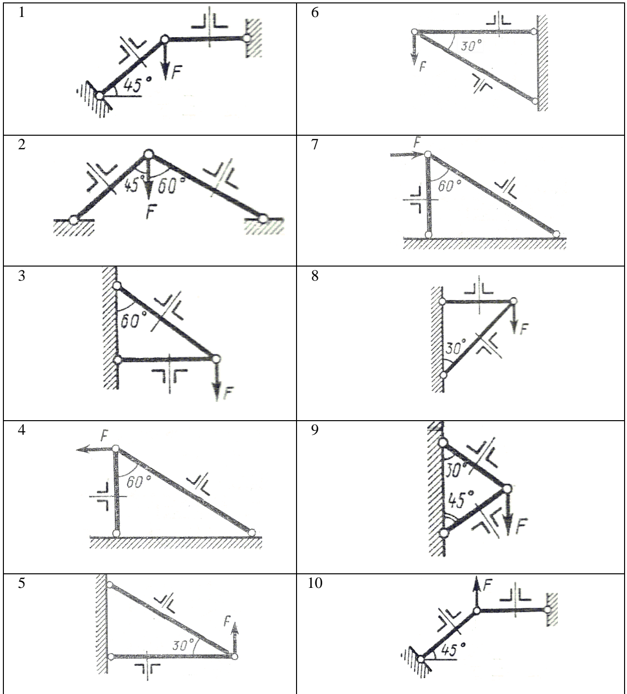
Рис. 9 - Схема задачи
