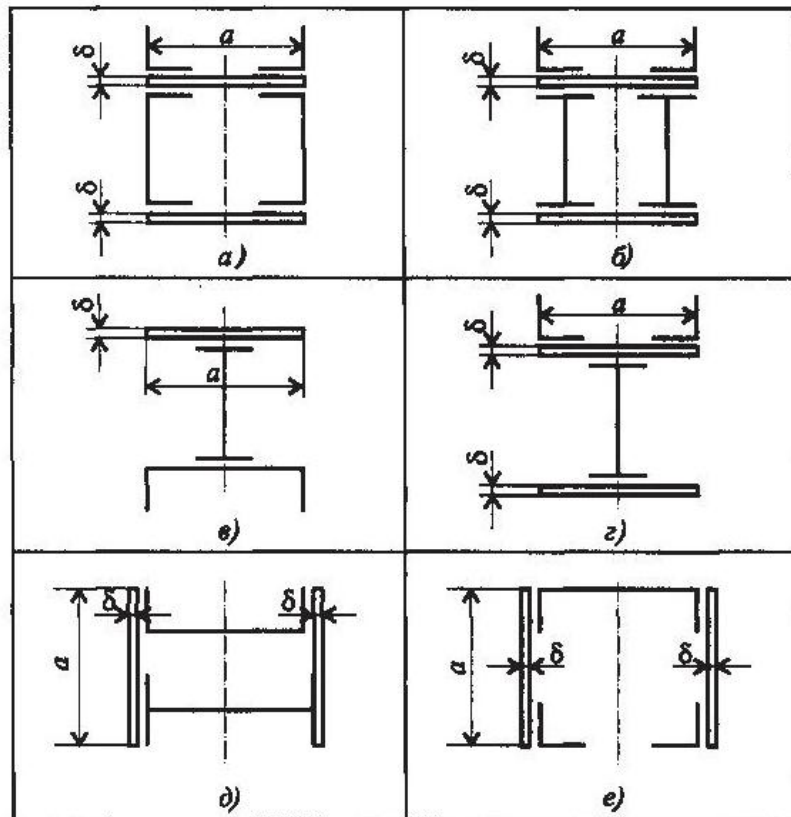
Рис.7 – Схема задачи
